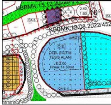
ÖNERİ PLAN
